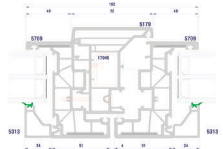
Sección horizontal
